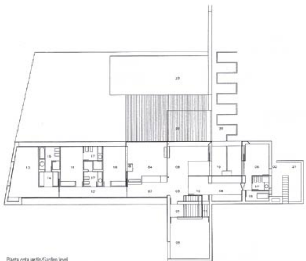
Planta cota jardín/Garden level
