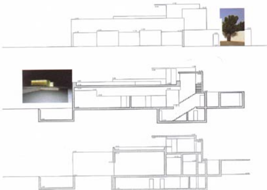
Secciones longitudinales por la fachada a naciente, por el núcleo de comunicaciones y por las estancias principales/ Longitudinal sections through the east façade, the communication nucleus and the main rooms
