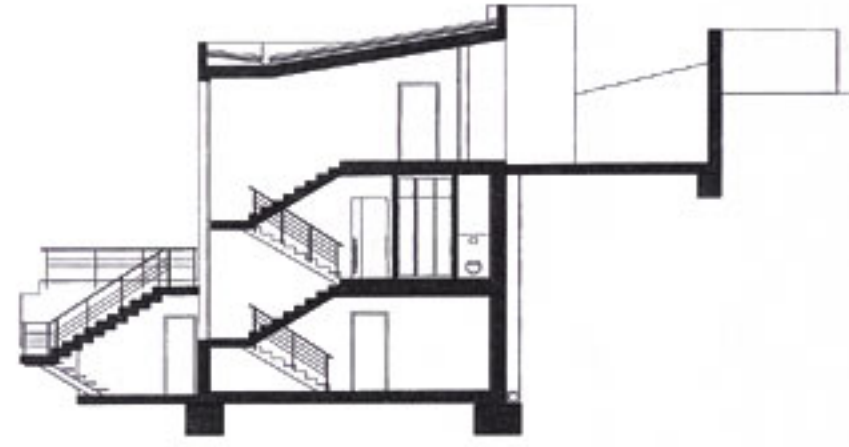
Sección B-B/Section BB
