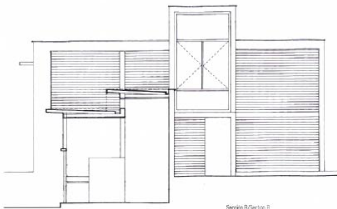
Sección B/Section B
