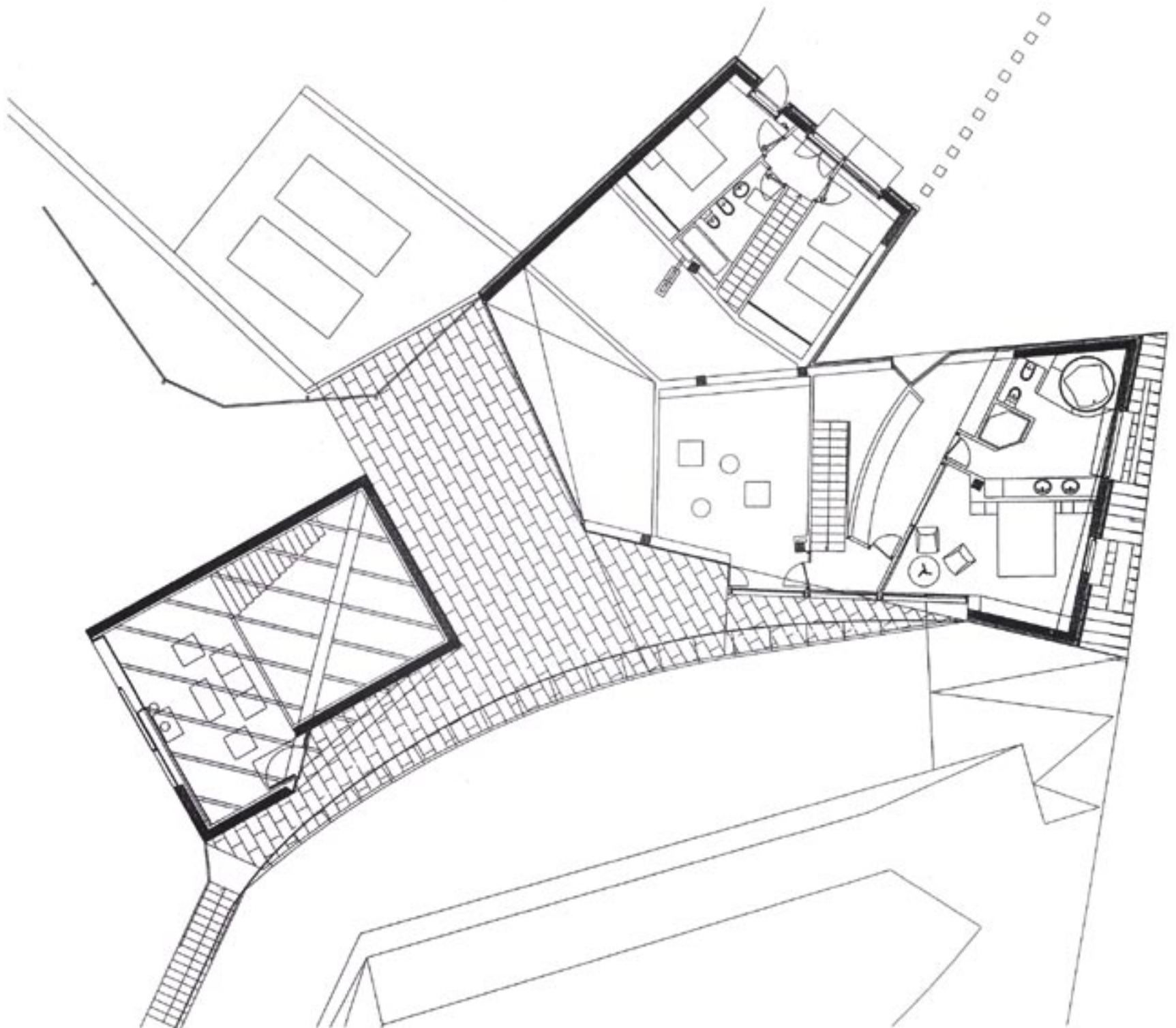
Planta primera/First floor
