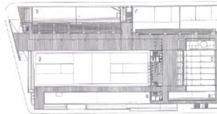
Planta baja/Ground floor
