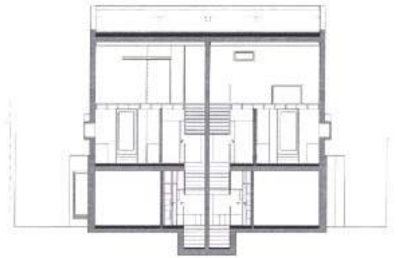
Sección A/Section A
